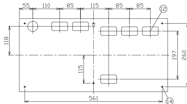
ケース底面ノックアウト図
