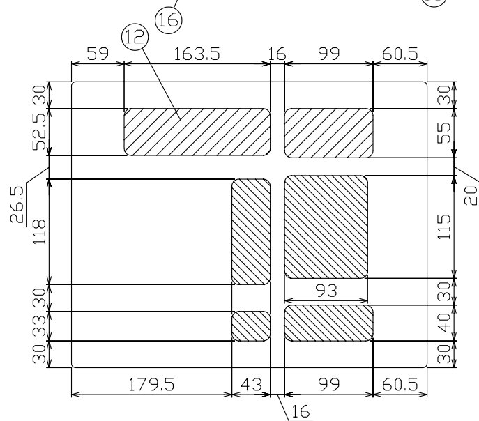
配線孔寸法図
