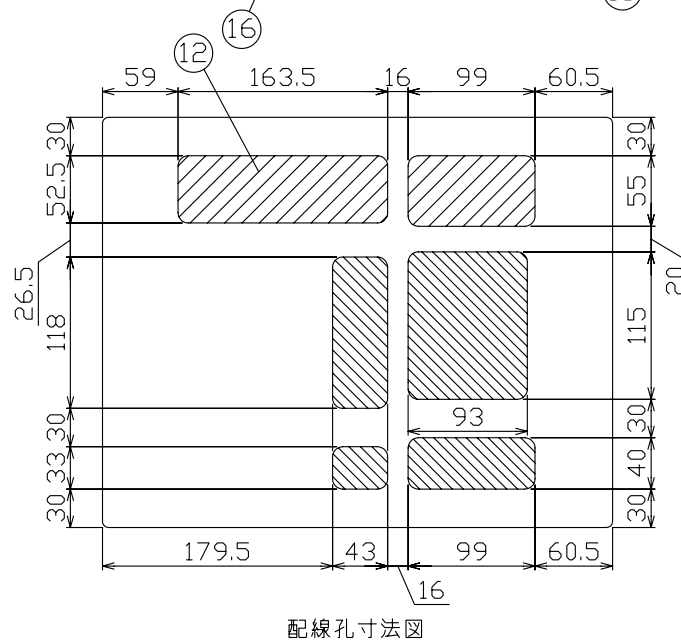
配線孔寸法図
