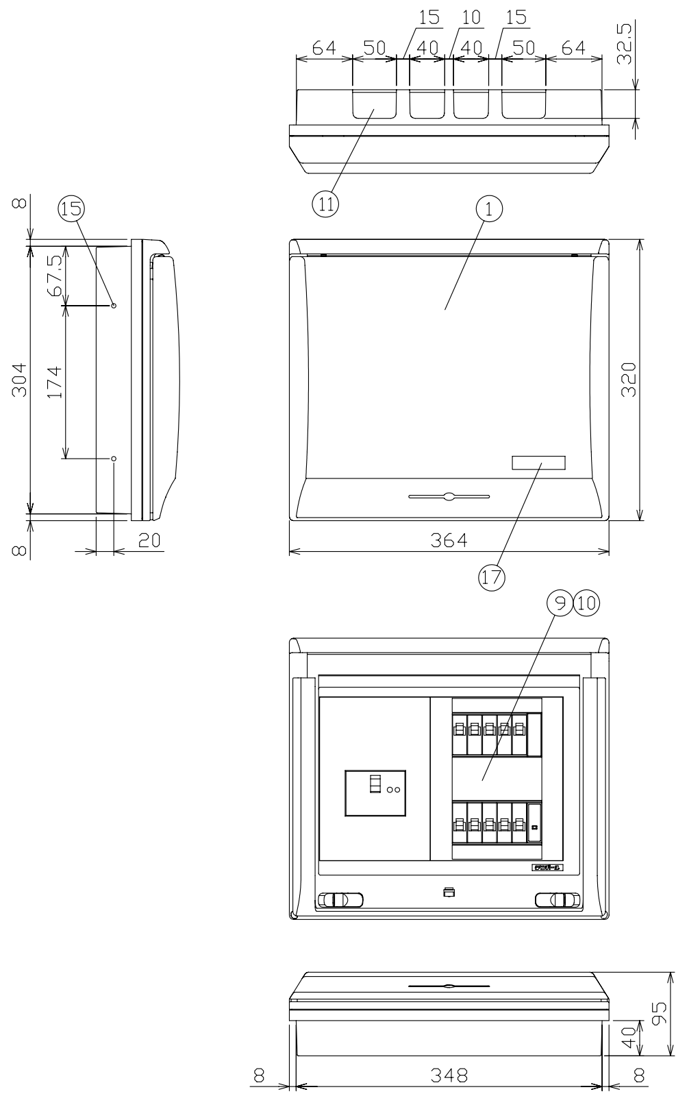
配線孔寸法図
