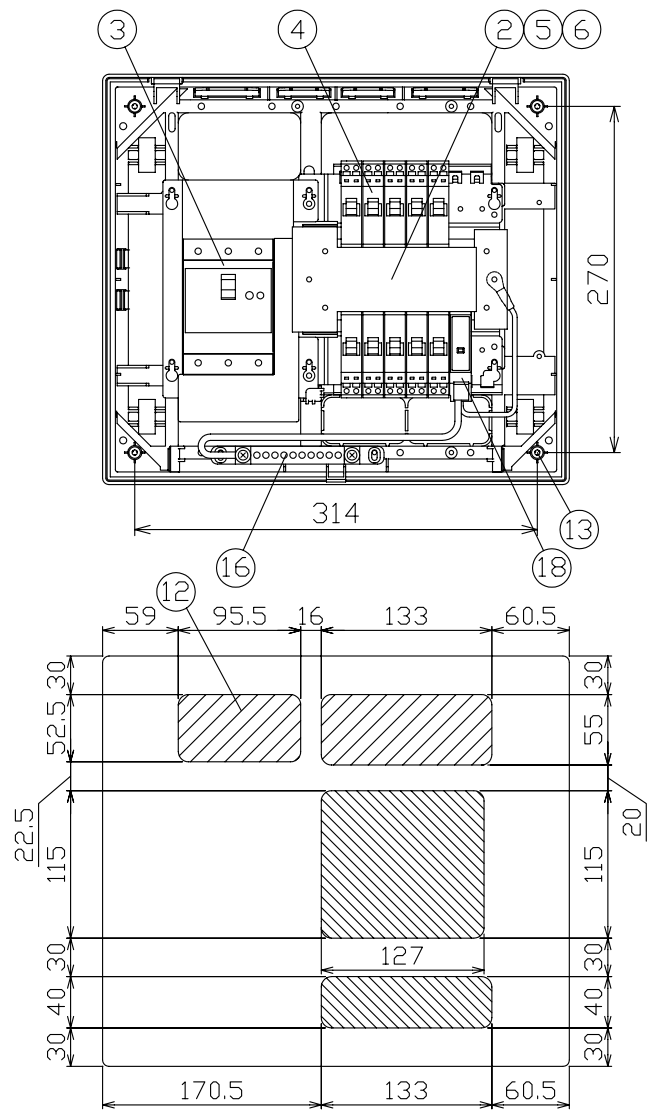
配線孔寸法図
