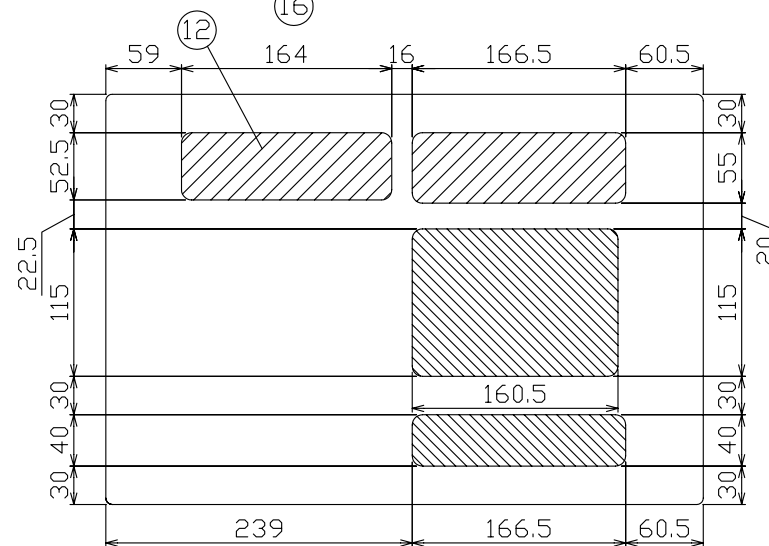
配線孔寸法図
