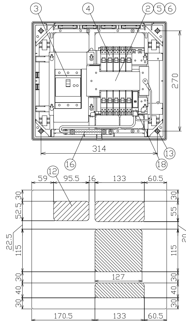
配線孔寸法図
