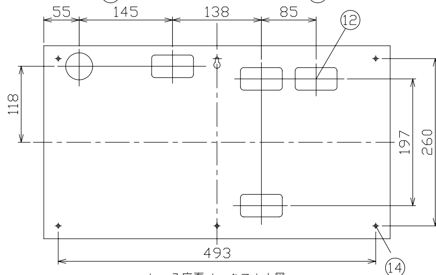
ケース底面ノックアウト図
