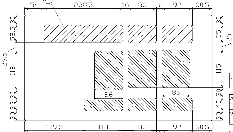
配線孔寸法図
