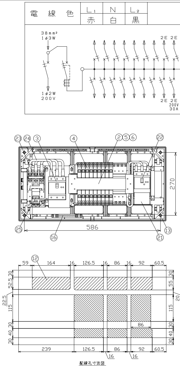
配線孔寸法図
