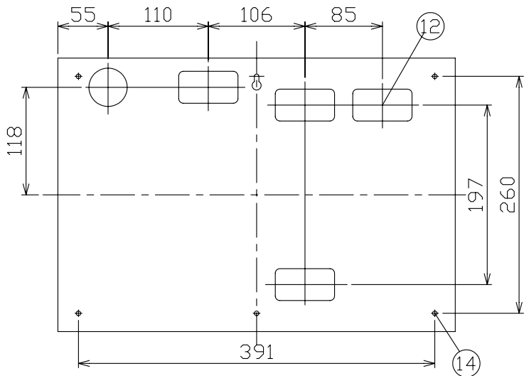
ケース底面ノックアウト図
