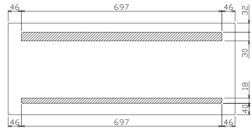
配線孔寸法図(////部開口)
