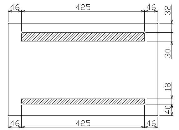
配線孔寸法図(////部開口)
