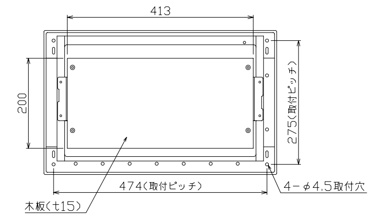
配線孔寸法図(////部開口)
