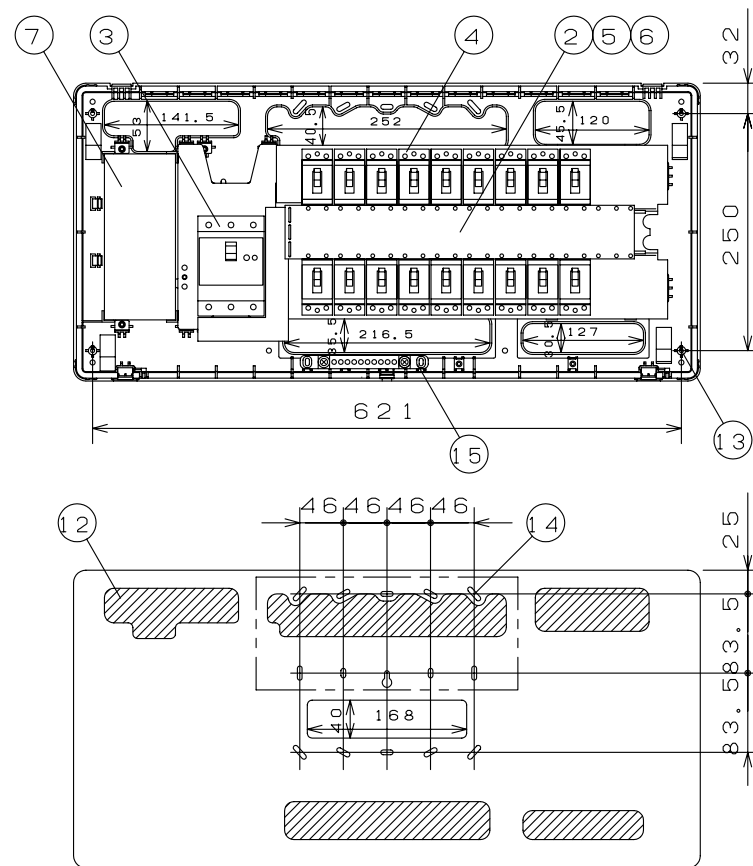
スイッチボックス位置図
