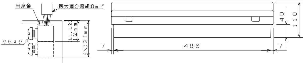
主幹用漏電遮断器端子構造
