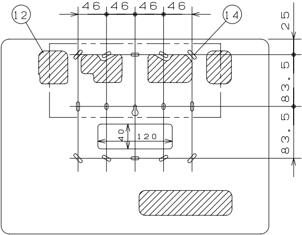
スイッチボックス位置図
