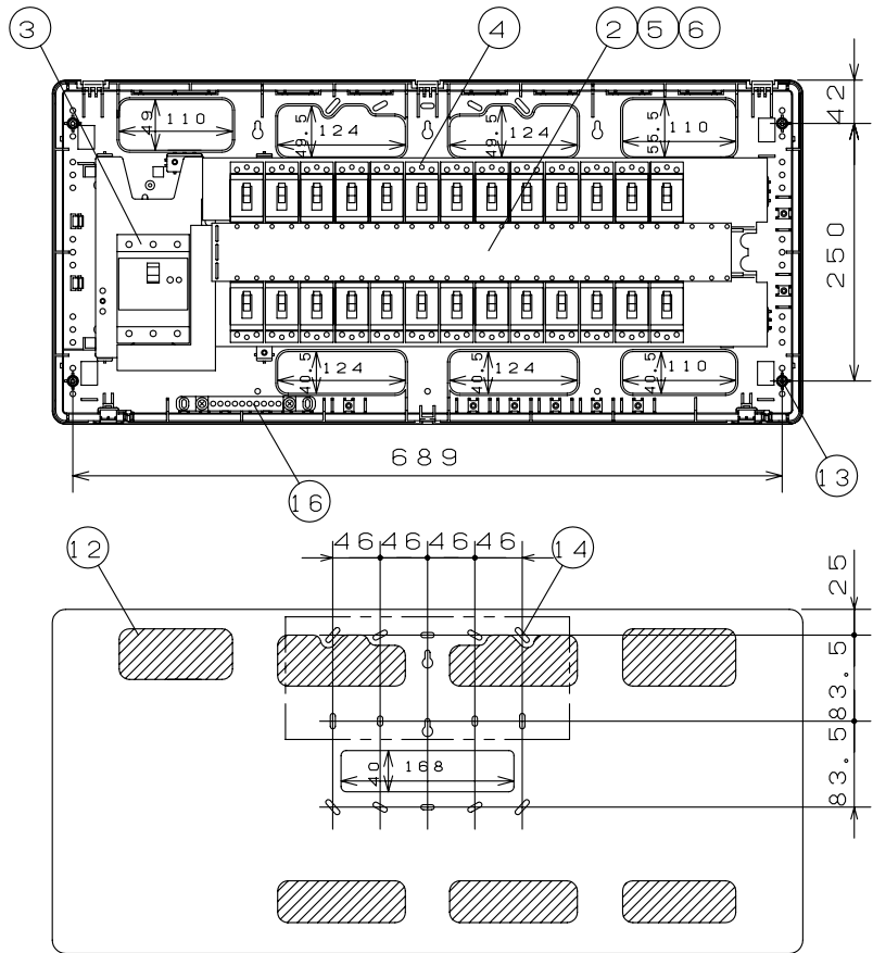
スイッチボックス位置図
