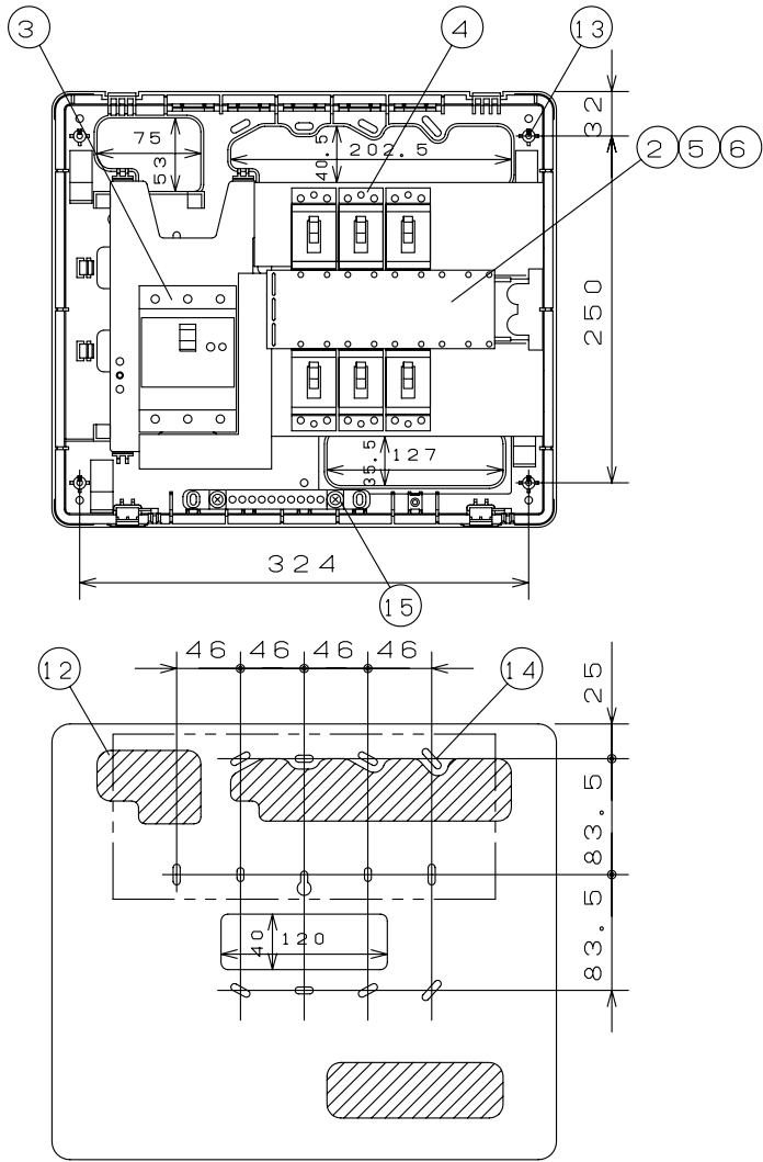
スイッチボックス位置図
