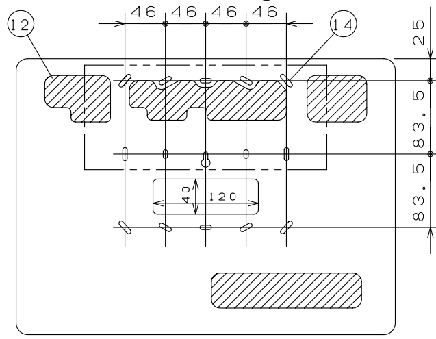
スイッチボックス位置図
