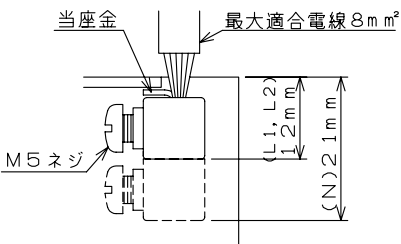
主幹用漏電遮断器端子構造
