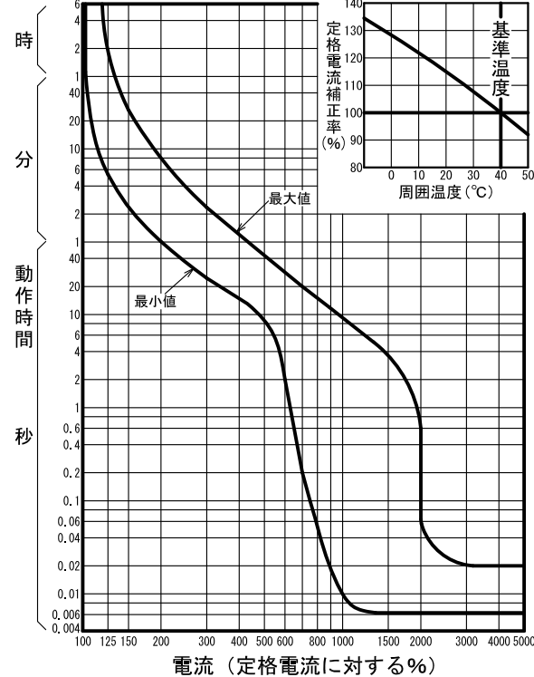
動作特性曲線
