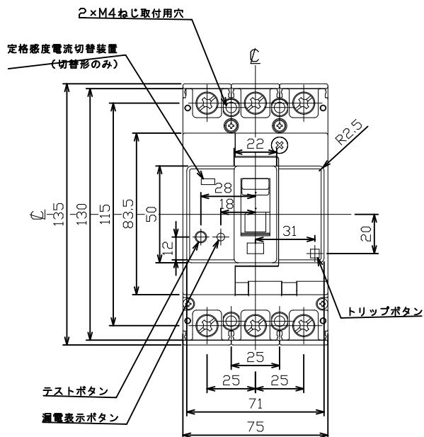
穴明寸法
