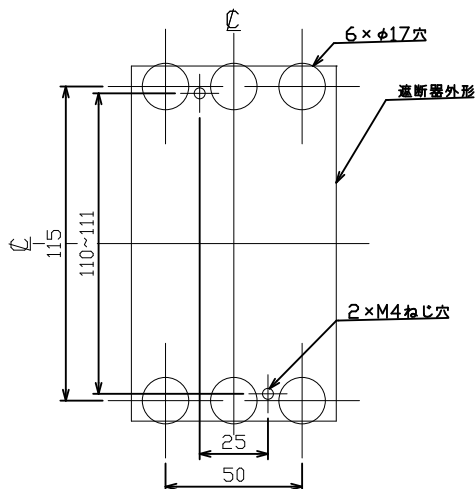
穴明寸法
