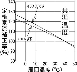
温度補正曲線
