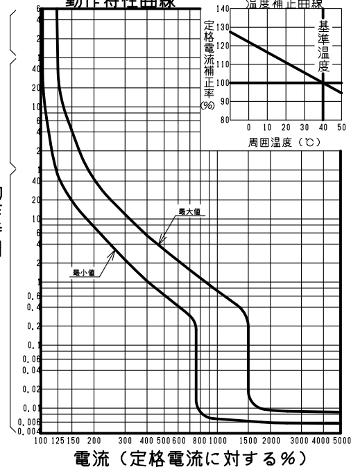
動作特性曲線
