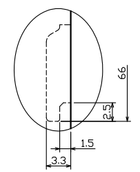
取付部 (A部) 詳細
