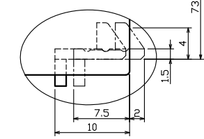
ロックレバー部 (B部) 詳細
