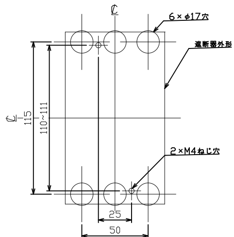
穴明寸法
