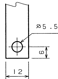
導線加工図
