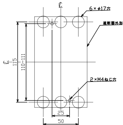
穴明寸法
