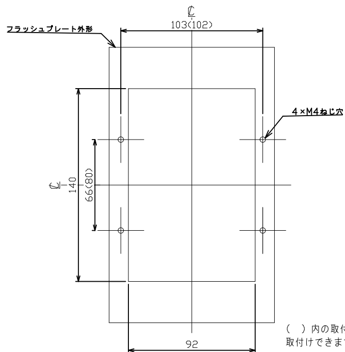
穴明寸法
