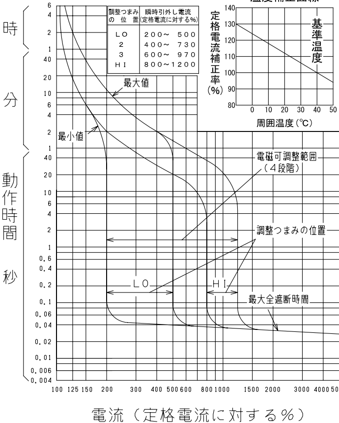
動作特性曲線
