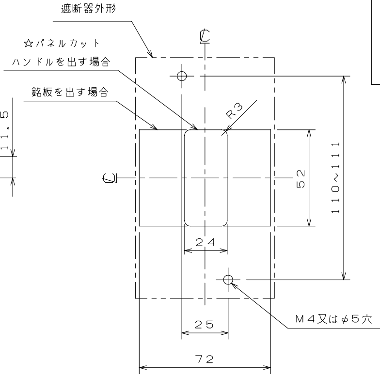
穴明寸法
