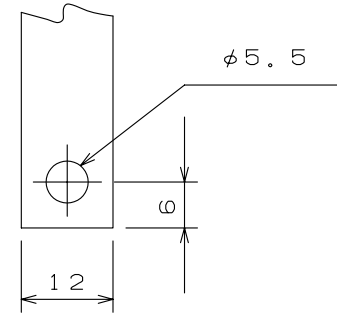
導帯加工図
