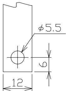
導帯加工図
