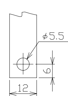
導帯加工図
