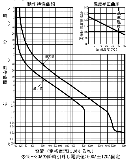
定格電流 15A, 20A, 30A
