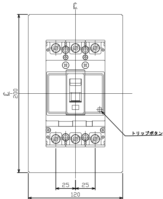
穴明寸法
