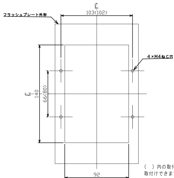
穴明寸法
