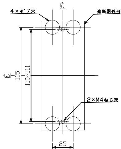
穴明寸法
