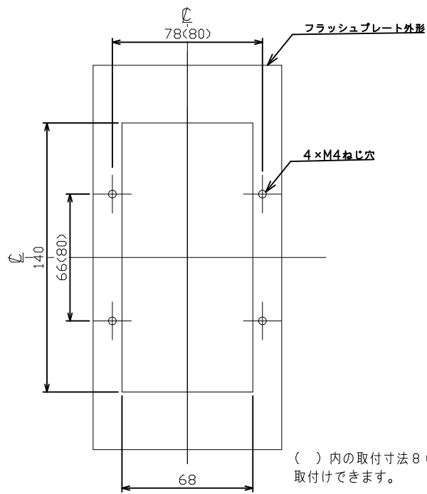
穴明寸法
