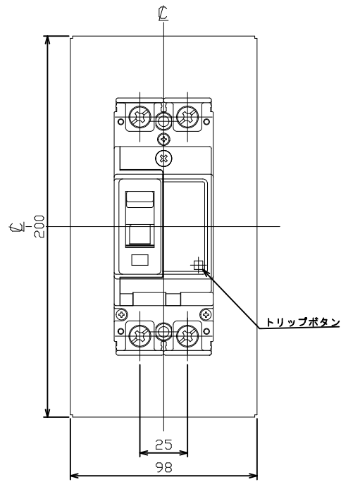
穴明寸法
