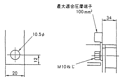
導帯加工図
