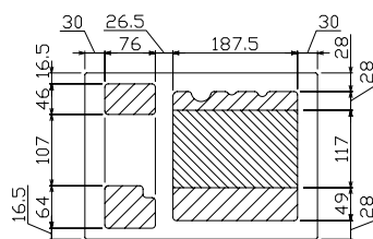
配線孔寸法図(//部開口, //部分岐背面)
