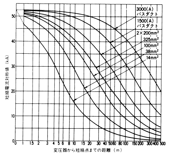
付図23 三相変圧器容量2000kVA、2次電圧415V
