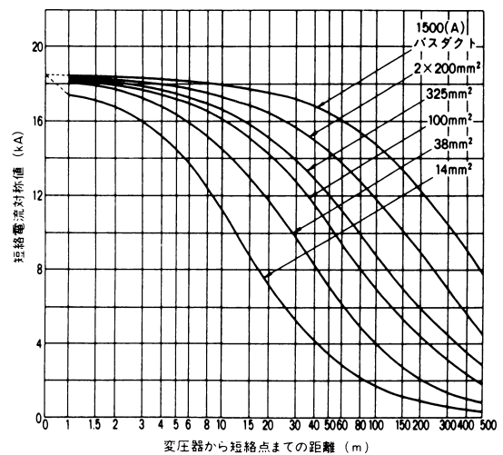
付図21 三相変圧器容量1500kVA、2次電圧415V
