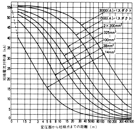
付図16 三相変圧器容量750kVA、2次電圧200V
