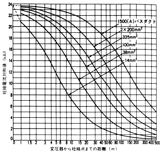
付図14 三相変圧器容量500kVA、2次電圧200V
