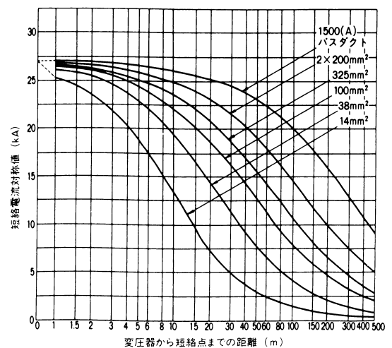
付図17 三相変圧器容量750kVA、2次電圧415V
