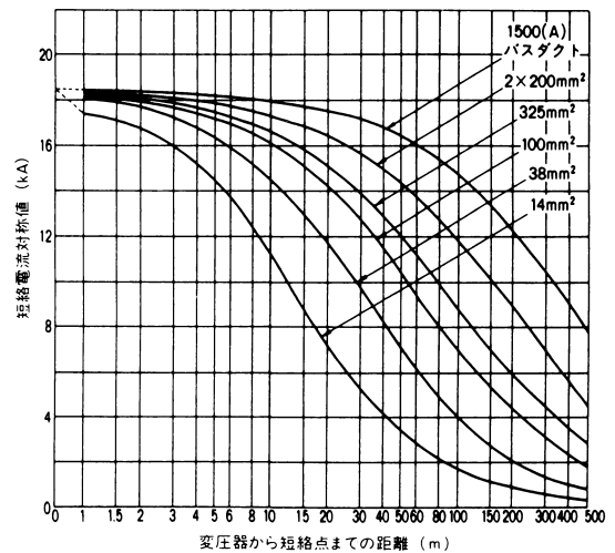
付図15 三相変圧器容量500kVA、2次電圧415V
