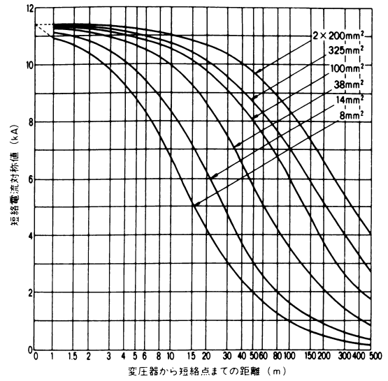
付図13 三相変圧器容量300kVA、2次電圧415V
