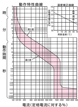
GB-53FKB(40A、50A)
