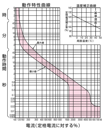
GB-53FKB(15A、20A、30A)
