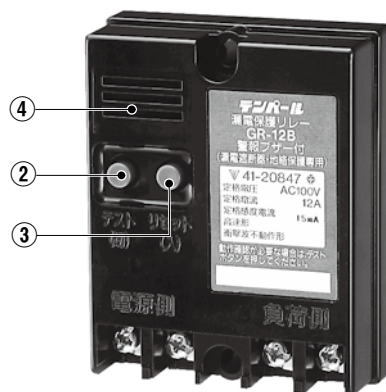
GR-12B (ブザー仕様)
