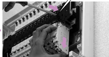
③指をA部に向け、ブレーカを引きながら、プラスドライバでB部を押し、ブレーカを取り外す。 *プラスドライバは、2番または3番。 *ブレーカの脱落に注意してください。
