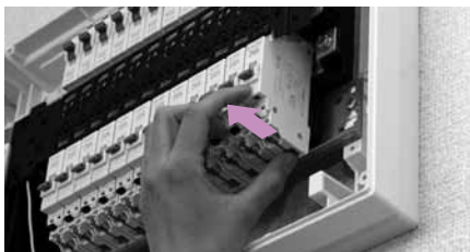
②ロックレバーを引き上げるようにスライドさせてロックを外す。
