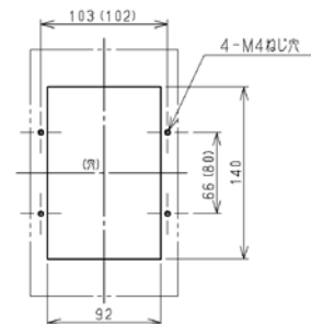
せん孔図
