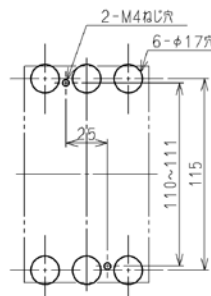
穴明寸法
