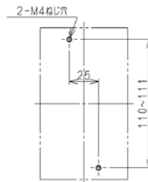
せん孔図
