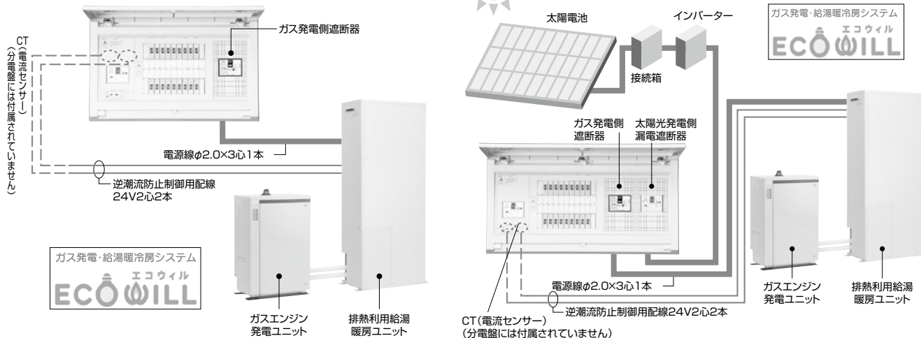
家庭用ガス発電・給湯暖房機用電気系統接続概要図
