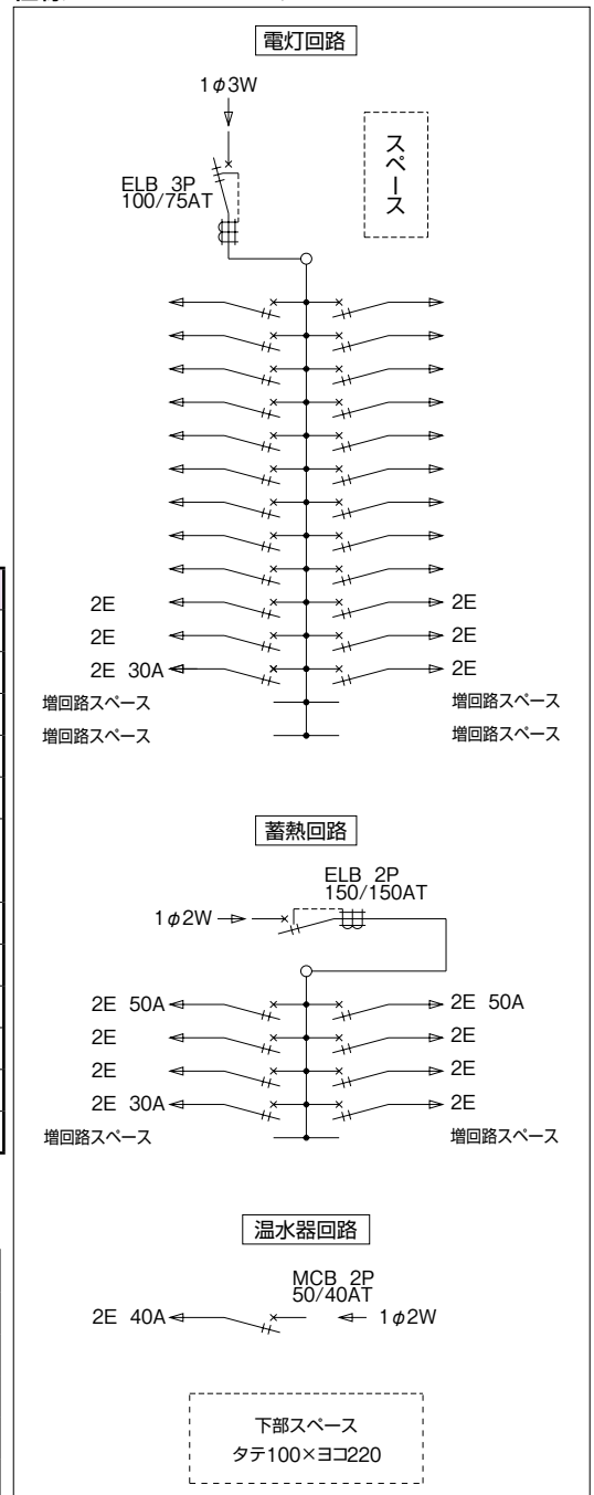
仕様 分岐：パールミニブレーカ ボックスサイズ/ H1,100×W400×D120 (スチール製)
