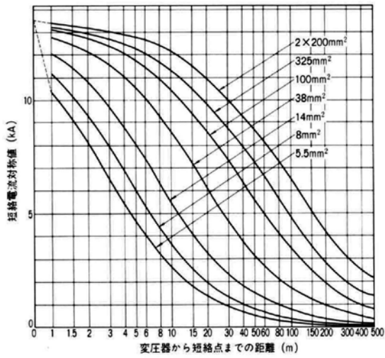
付図30 単相3線式変圧器容量150kVA、外線間200V
