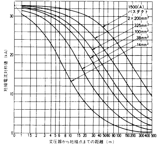
付図19 三相変圧器容量1000kVA、2次電圧415V
