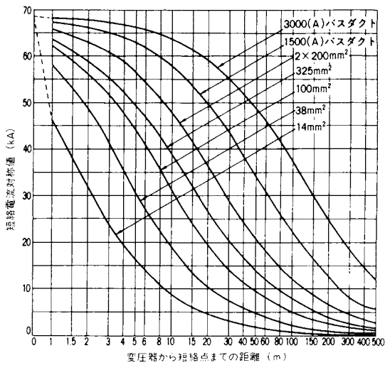
付図20 三相変圧器容量1500kVA、2次電圧200V
