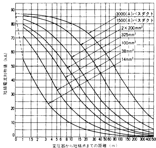
付図22 三相変圧器容量2000kVA、2次電圧200V
