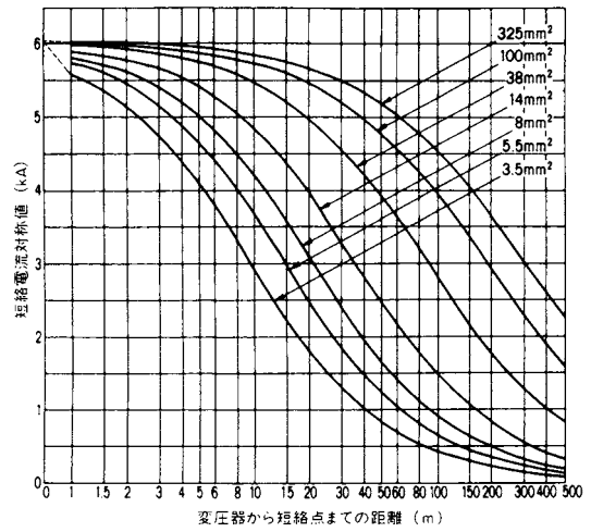
付図7 三相変圧器容量100kVA、2次電圧415V
