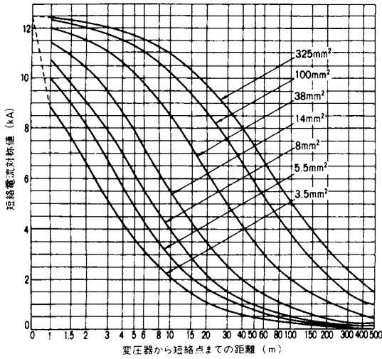
付図8 三相変圧器容量150kVA、2次電圧200V
