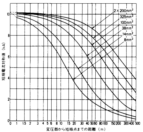
付図11 三相変圧器容量200kVA、2次電圧415V
