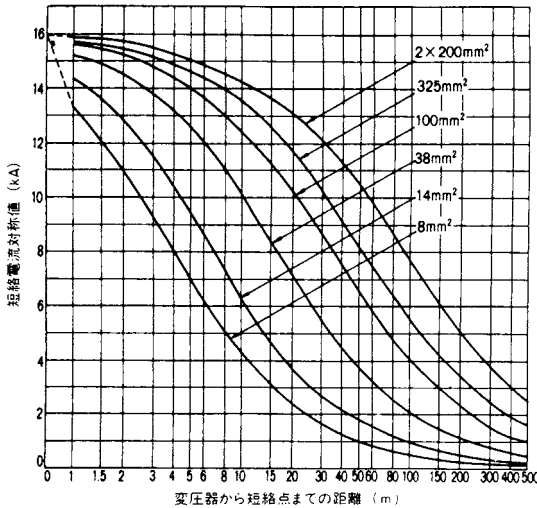
付図10 三相変圧器容量200kVA、2次電圧200V
