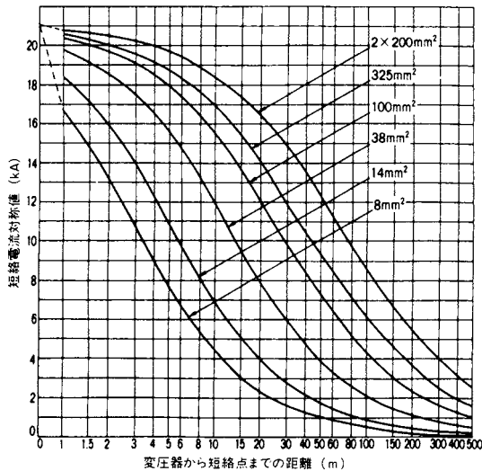
付図10 三相変圧器容量200kVA、2次電圧200V
