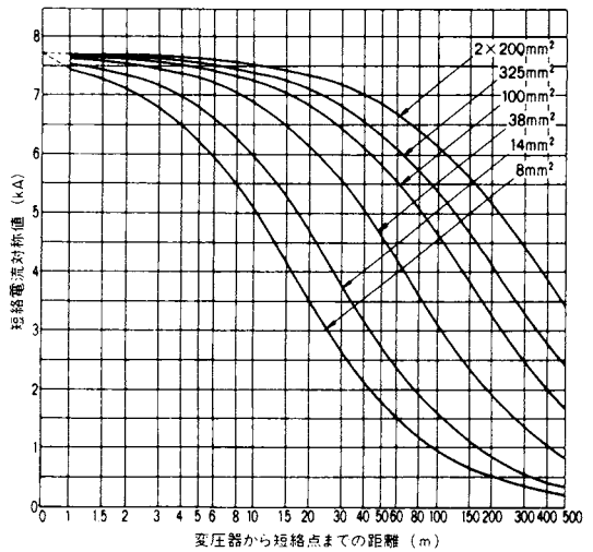
付図11 三相変圧器容量200kVA、2次電圧415V
