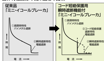
動作特性曲線の従来品との比較
