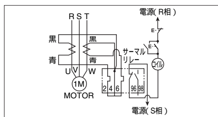
サーマルリレーとCTの結線図
